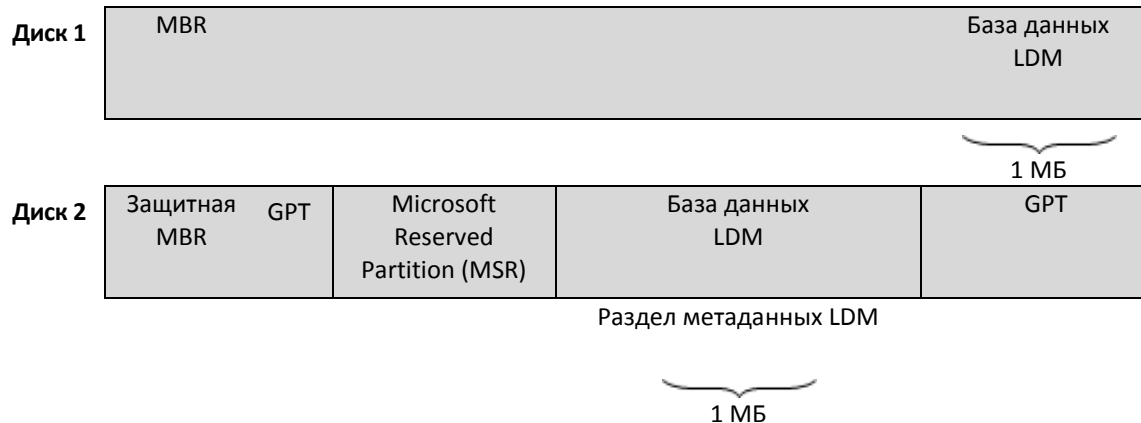
Динамический MBR-диск (Диск 1) и динамический GPT-диск (Диск 2).
